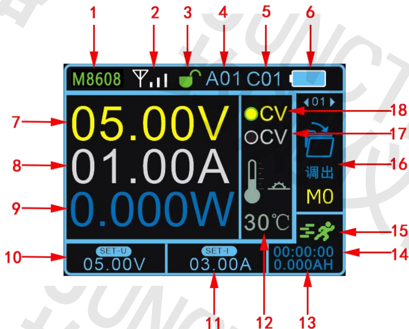
图 2-3-1 DPM8600 系列数控电源无线控制器图示
