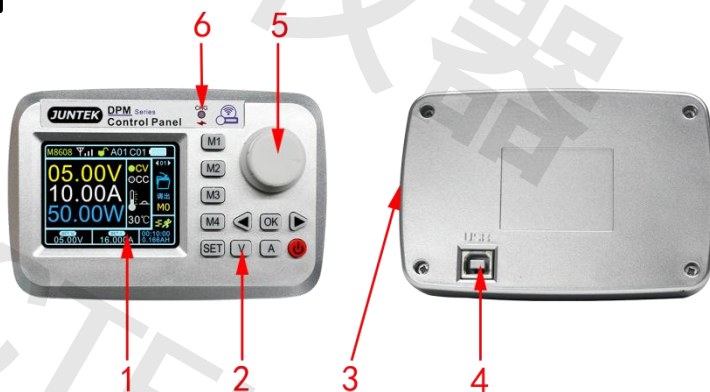
图 2-2-1 DPM8600 系列数控电源无线控制器图示
