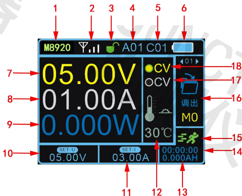
图 2-3-1 DPH8900 系列数控电源无线控制器图示
